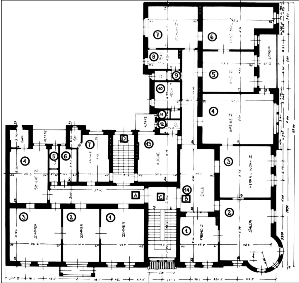
2. Projekt rzutu pierwszego piętra kamienicy mieszczańskiej przy ul. Rutgerstrasse 9 w Katowicach (1908 r.), w: M. Krysiak, W kamienicy mieszczańskiej , Chorzów, b. r., s. 18. Plan przedstawia mieszkanie małe (A) i duże (B), podzielone klatką schodową. W części A łazienka znajduje się przy sypialni państwa (4) a klozet pod nr 5; w części B łazienka umieszczona pod nr 8 a klozet nr 9
