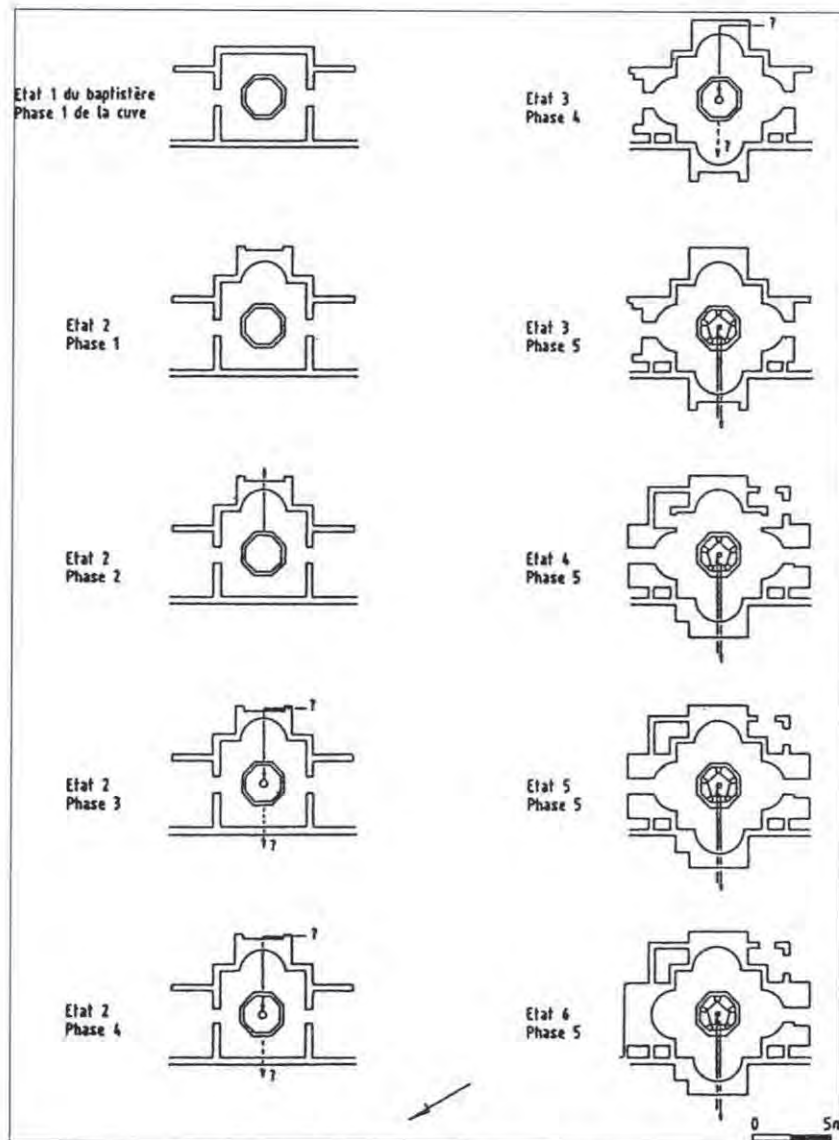
8. Grenoble. Baptysterium. Plan (kolejne fazy)
