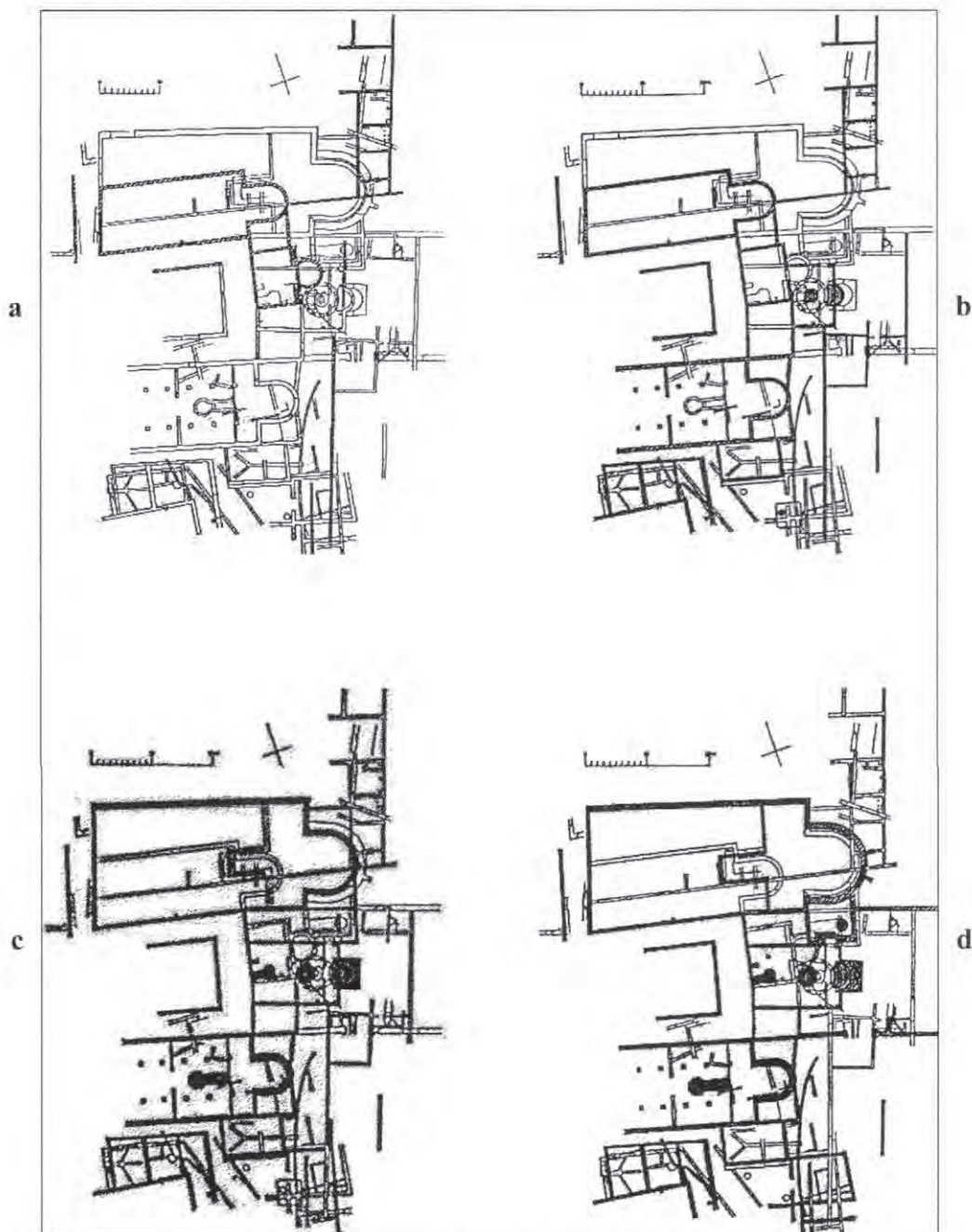
7. Genewa. Zespól biskupi. Plany (a – 2. poł. IV w.; b – ok. 400 r.; c – V w.; d – VI w.)
