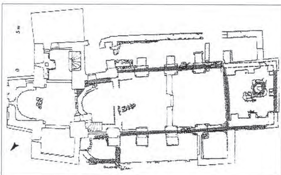
3. Châteauneuf-de-Grasse. Kościół Notre-Dame du Brusse. Plan
