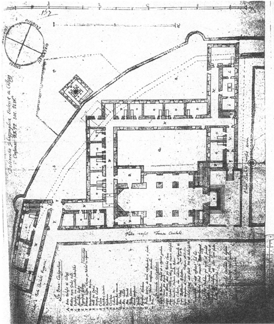
2. Plan kościoła i klasztoru Jezuitów w Krosnie, 1697 ?/, Bibliothèque Nationale de Paris, wg Vallery-Radot, s. 326
