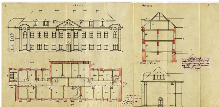
3. K. Srokowski, projekt przebudowy oficyny przy zamku w Białej Podlaskiej, 1923. Archiwum Państwowe w Lublinie, Urząd Wojewódzki Lubelski 1919-1939, Wydział Komunikacyjno-Budowlany, sygn. 414. Fot. Pracownia Reprograficzna Archiwum Państwowego w Lublinie
