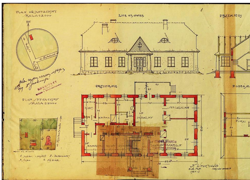
2. K. Srokowski, projekt plebanii w Kornicy, 1924. Archiwum Państwowe w Lublinie, Urząd Wojewódzki Lubelski 1919-1939, Wydział Komunikacyjno-Budowlany, sygn. 1123. Fot. Pracownia Reprograficzna Archiwum Państwowego w Lublinie
